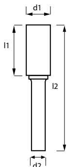
Размеры — все в мм | Номера деталей
